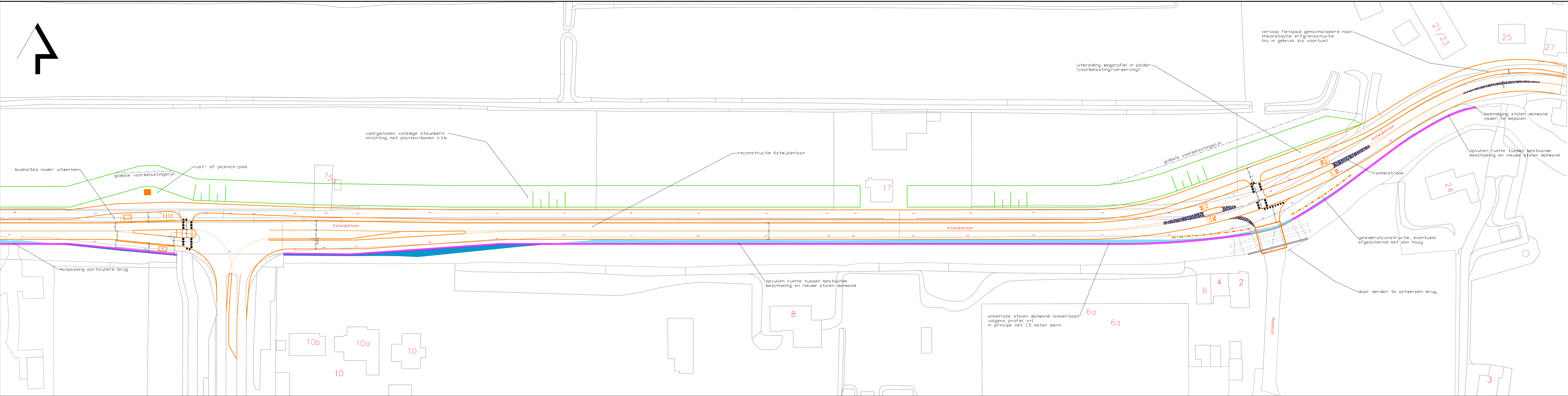
SITUATIE TUSSEN KATWIJKERLAAN 10 EN KATWIJKERLAAN 27
