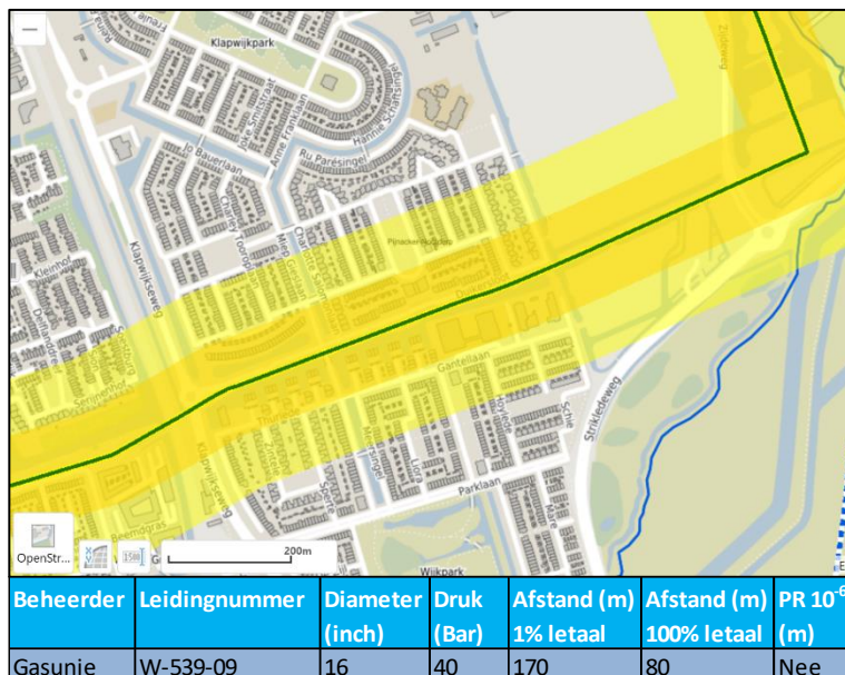
Overzicht ligging en eigenschappen aardgastransportleiding.
