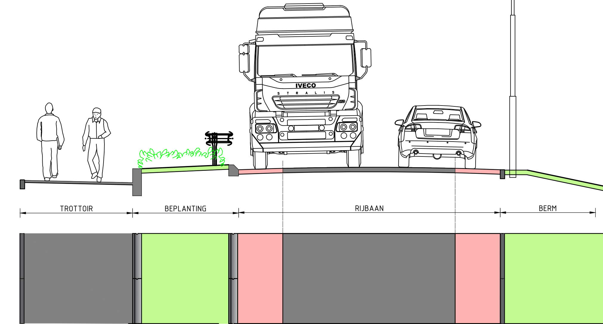
Profiel t.p.v. kruispunt (Katwijkerlaan)
