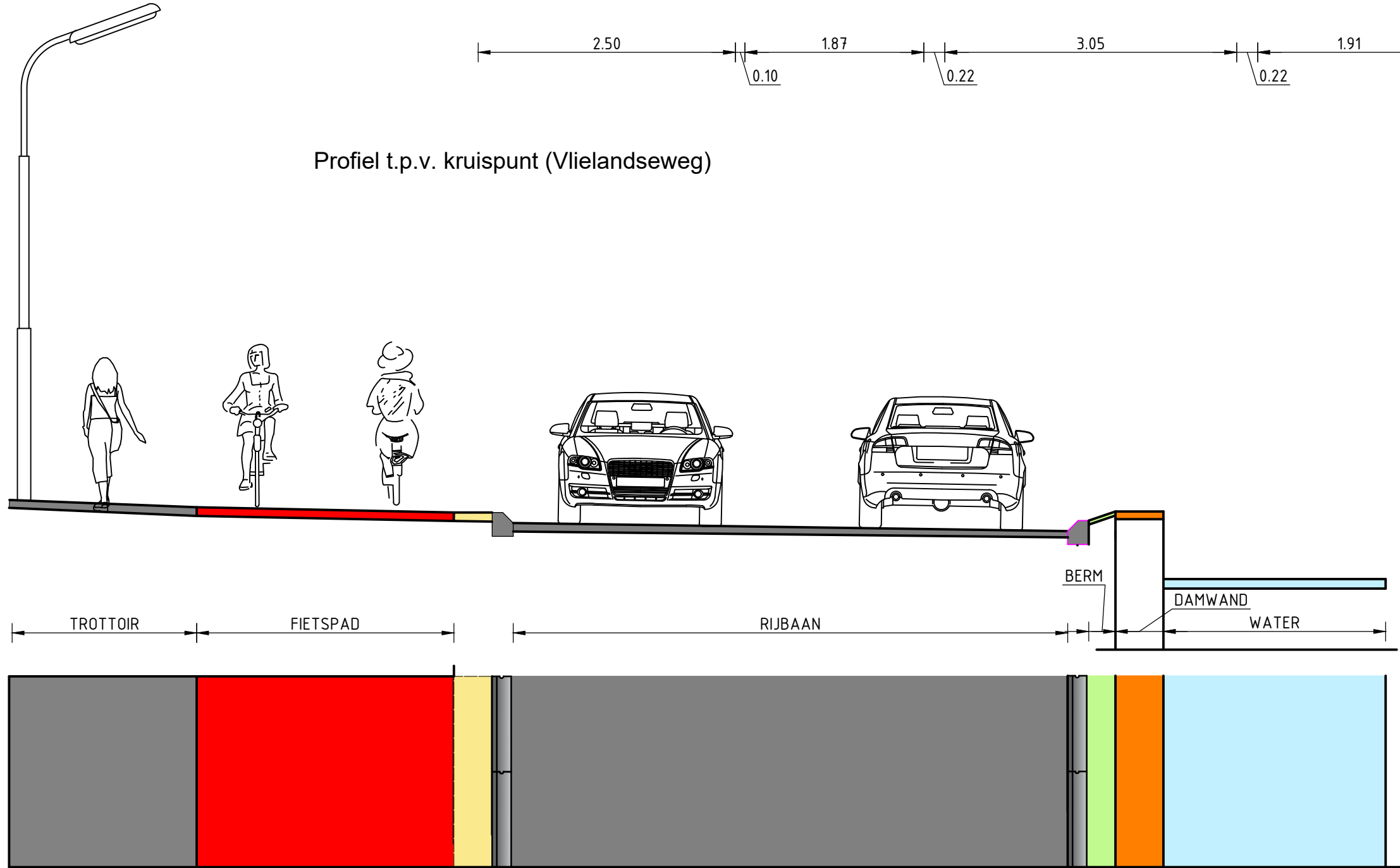
Profiel t.p.v. Vlielandseweg
