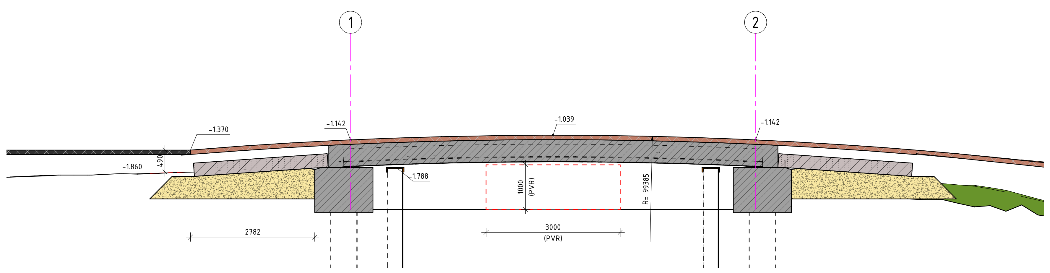
LANGSDOORSNEDE schaal: 1 : 50
