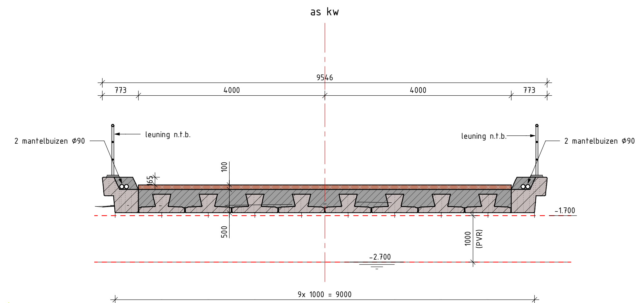
DWARSDOORSNEDE schaal: 1 : 50
